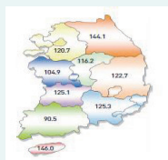
임목축적
