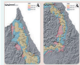
백두대간 수치지도
