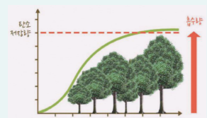
산림탄소흡수량 산정
