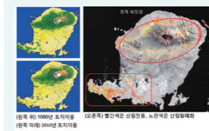
룸복의 산림전용 및 황폐화 지도(1990~2010)
