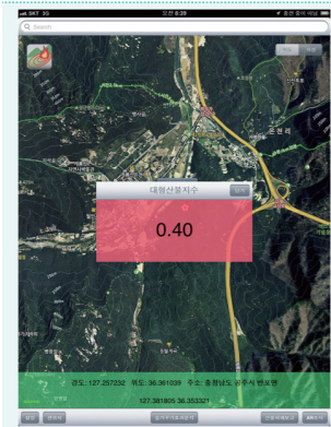
대형산불판정프로그램
