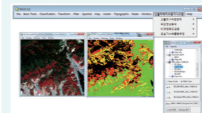
산불피해평가 시스템
